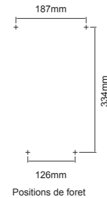
Montage horizontal
